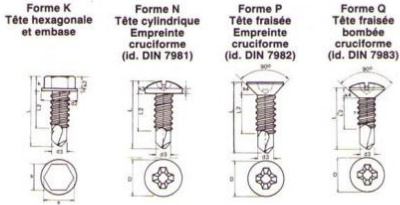
DIN 7504
