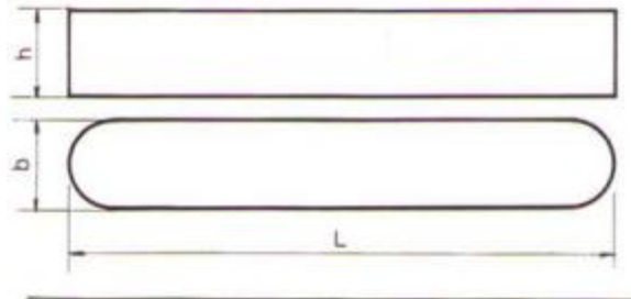
DIN 6885
