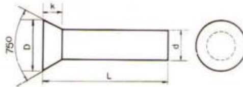
DIN 661
