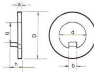
DIN 462
