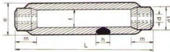
DIN 1480
